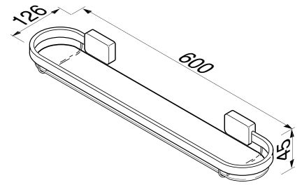
917001 Planchet 60 cm Shelf holder 60 cm Abstellgarnitur 60 cm Étagère 60 cm Repisa 60 cm
