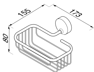
912714-02 Fles- en sponshouder Bottle/sponge holder Universalkorb Corbeille universelle Combinación de Canasta
