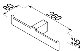
913518-02 Toiletrolhouder, dubbel Toilet roll holder, double Toilettenpapierhalter, doppelt Porte-papier rouleau, double Portarollos, doble
