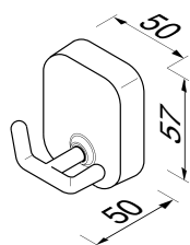
912415-02 Haak, dubbel Hook, double Haken, doppelt Porte-peignoir/crochet, double Gancho, doble
