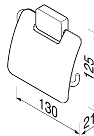
917008 Toiletrolhouder Toilet roll holder Toilettenpapierhalter Porte-papier rouleau Portarollos
