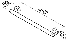
915807-02-45 Veiligheidsgreep 45 cm Safety grip handle 45 cm Sicherheitsgriff 45 cm Poignée de sécurité 45 cm Asidero de seguridad 45 cm
