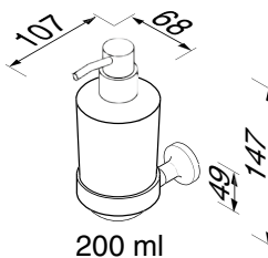
G 917316-02 Zeepdispenser 200 ml Soap dispenser 200 ml Seifenspender 200 ml Distributeur de savon 200 ml Dosificador de jabón 200 ml
