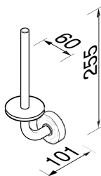
915518 Reserverolhouder, dubbel Spare roll holder, double Reserverollenhalter, doppelt Porte-papier rouleau de réserve, double Portarrollos de reserva doble
