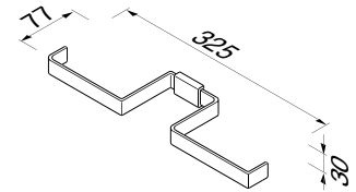
918418-02 Toiletrolhouder, dubbel Toilet roll holder, double Papierrollenhalter, doppelt Porte-papier rouleau, double Portarrollos, doble
