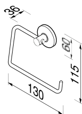
915309-02 Toiletrolhouder Toilet roll holder Porte-papier rouleau Papierrollenhalter Portarrollos
