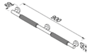
915807-62-90 Veiligheidsgreep 90 cm Safety grip handle 90 cm Sicherheitsgriff 90 cm Poignée de sécurité 90 cm Asidero de seguridad 90 cm
