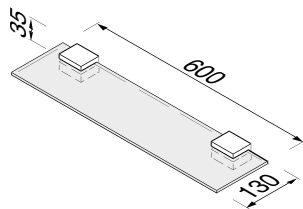
917545-02 Planchet 60 cm Shelf holder 60 cm Abstellgarnitur 60 cm Étagère 60 cm Repisa 60 cm
