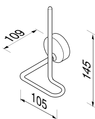
912712-02 Reserverolhouder Spare roll holder Reserverollenhalter Porte-papier rouleau de réserve Portarollos de reserva
