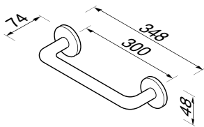
916574-02 Badgreep 30 cm Grab rail 30 cm Wannengriff 30 cm Poignée de bain 30 cm Manillón 30 cm
