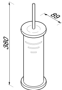
915116 Toiletborstelhouder, vrijstaand Toilet brush holder, free standing WC-Bürstengarnitur, Standmodell Porte-balai à poser Escobillero de pie
