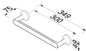
917306-04 Badgreep 30 cm Grab rail 30 cm Wannengriff 30 cm Poignée de bain 30 cm Manillón 30 cm
